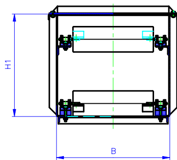
Snitt A-A Typ: TKF... L & LB
