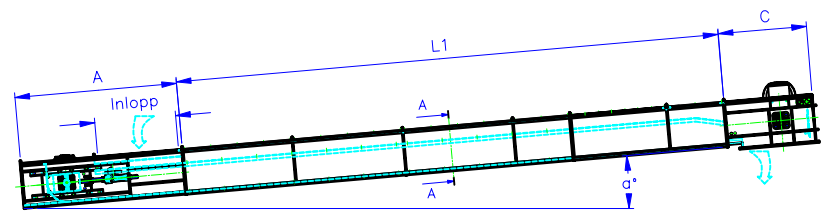
Typ TKF... L
